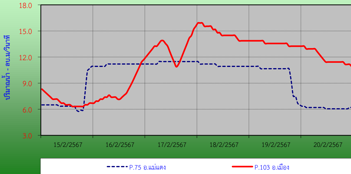
กราฟแสดงปริมาณน้ำปิ้งรายชั่วโมงรอบวันที่ 7/2567 ที่สถานีแม่ น้ำปิ้ง ( P.75) บ้านซ้อแล อ.แม่แตง และที่สถานีแม่ น้ำปิ้ง (P.103) บ้านป่าซ้อยใต้ อ.เมือง จ.เชียงใหม่
